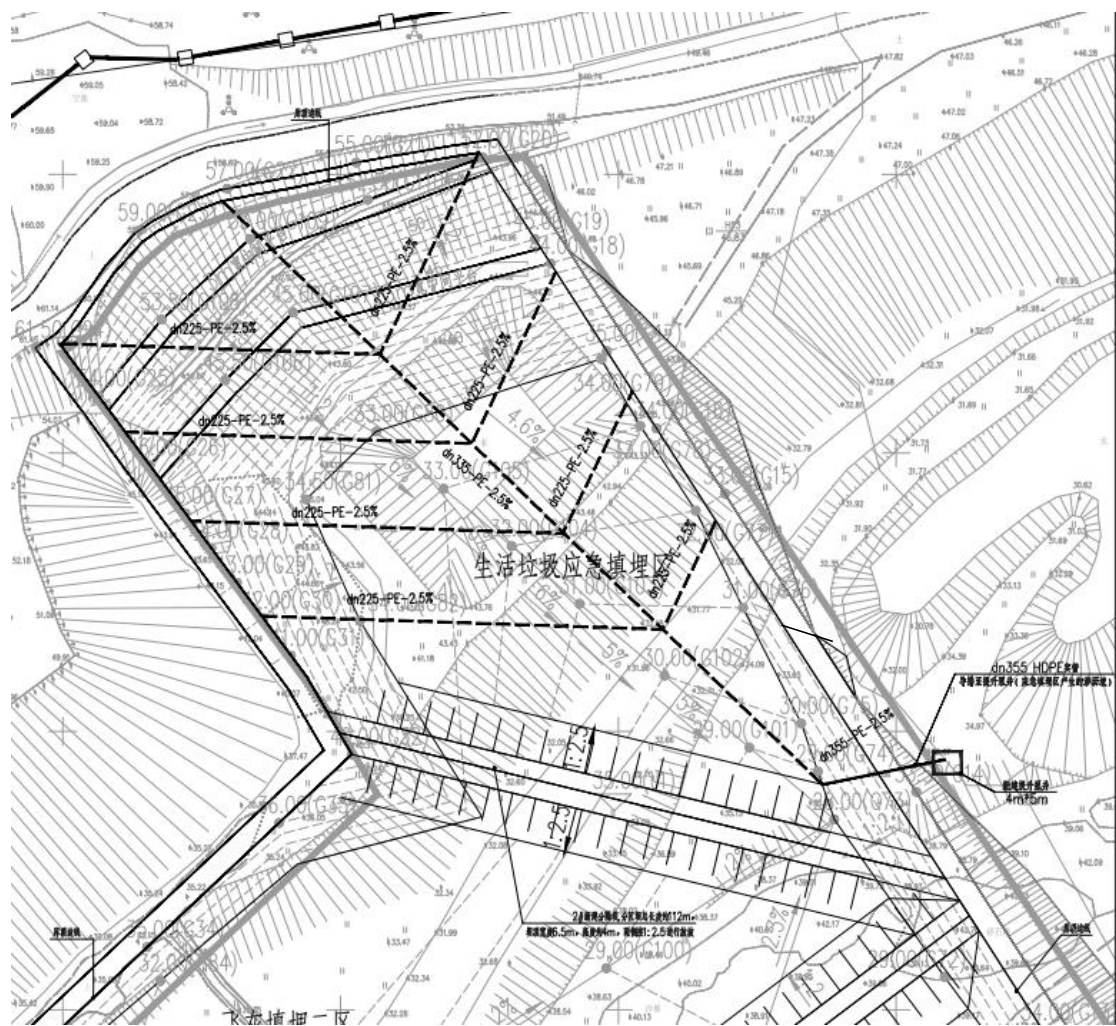
图 7.3-7 应急填埋区渗沥液收集系统平面图
